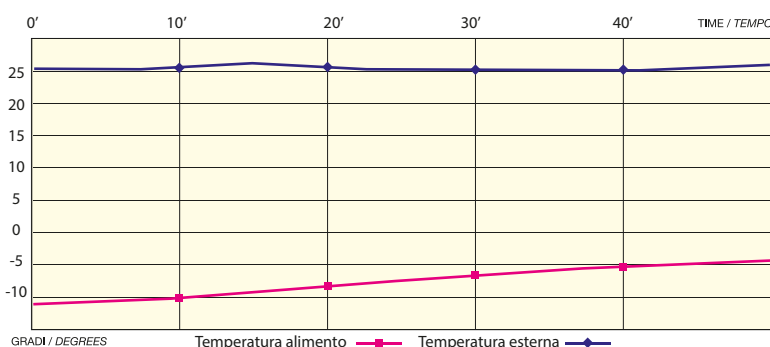
Prova di dispersione termica della vaschetta Ecogel
