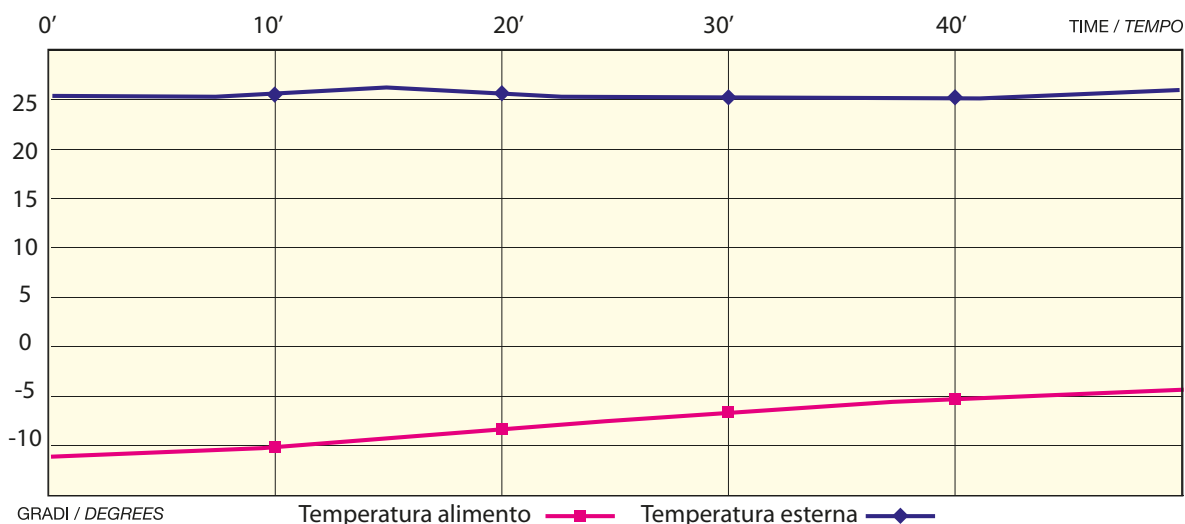
Prova di dispersione termica della vaschetta Ecogel
